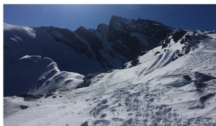
Corral del Veleta 1-2-17
