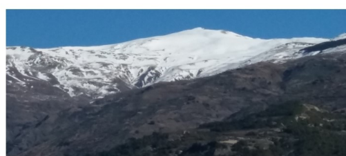
Tajos de la Virgen, Cartujo y Caballo 1-2-17
