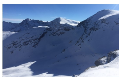
Corral del Veleta 1-2-17
