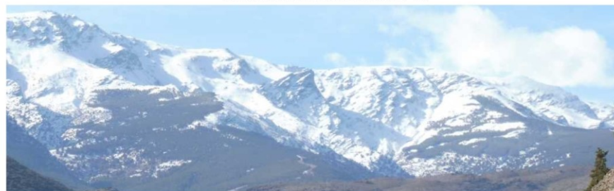
Cara norte cumbres almerienses 31-1-17
