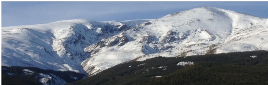
Picón de Jerez 1-2-17
